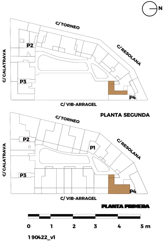
Portal 4. Vivienda 1 Planta primera y segunda
