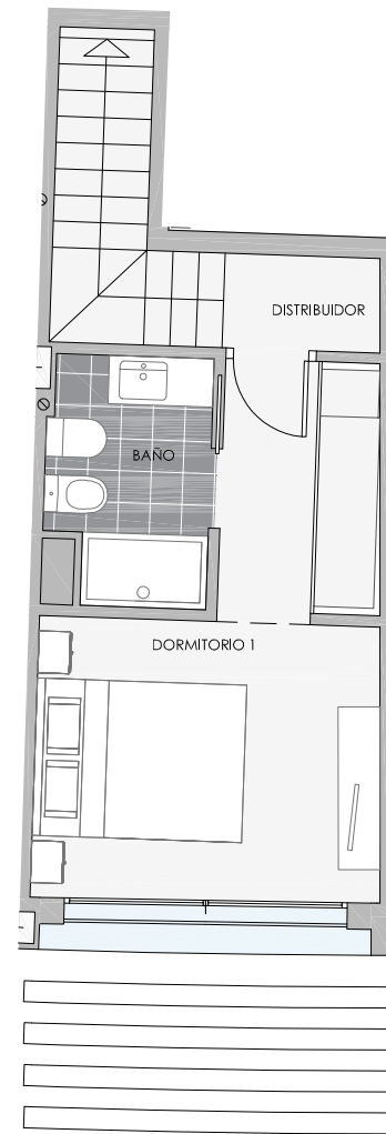
PLANTA PRIMERA
