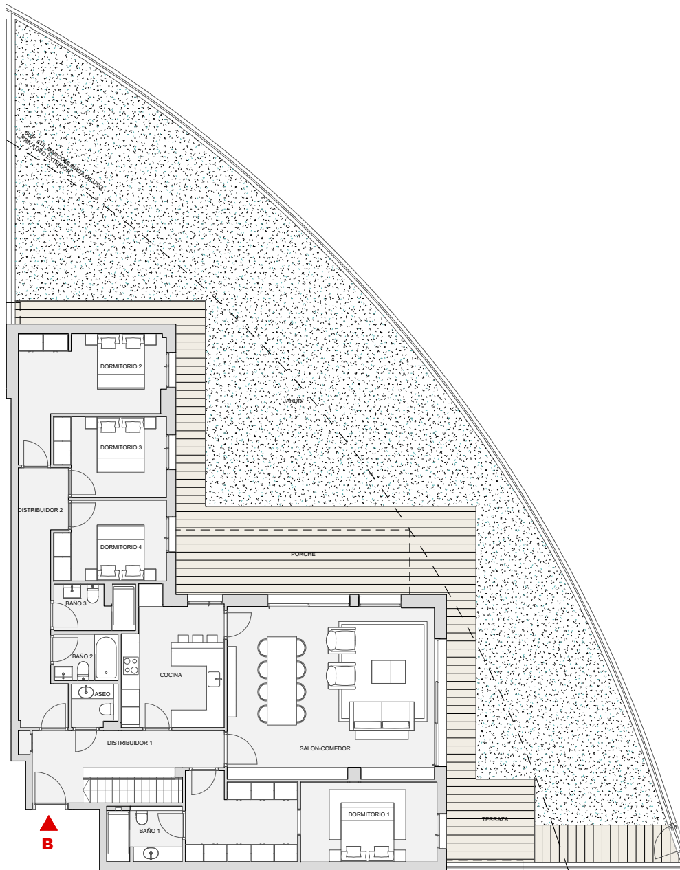
PLANTA BAJA
