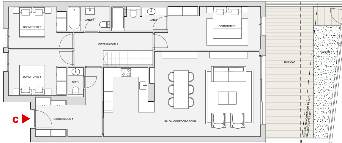
PLANTA BAJA
