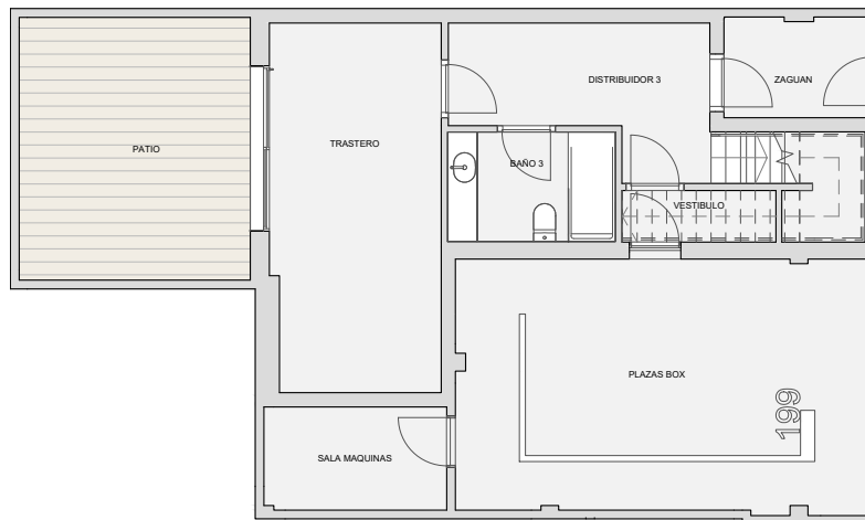
PLANTA SÓTANO
