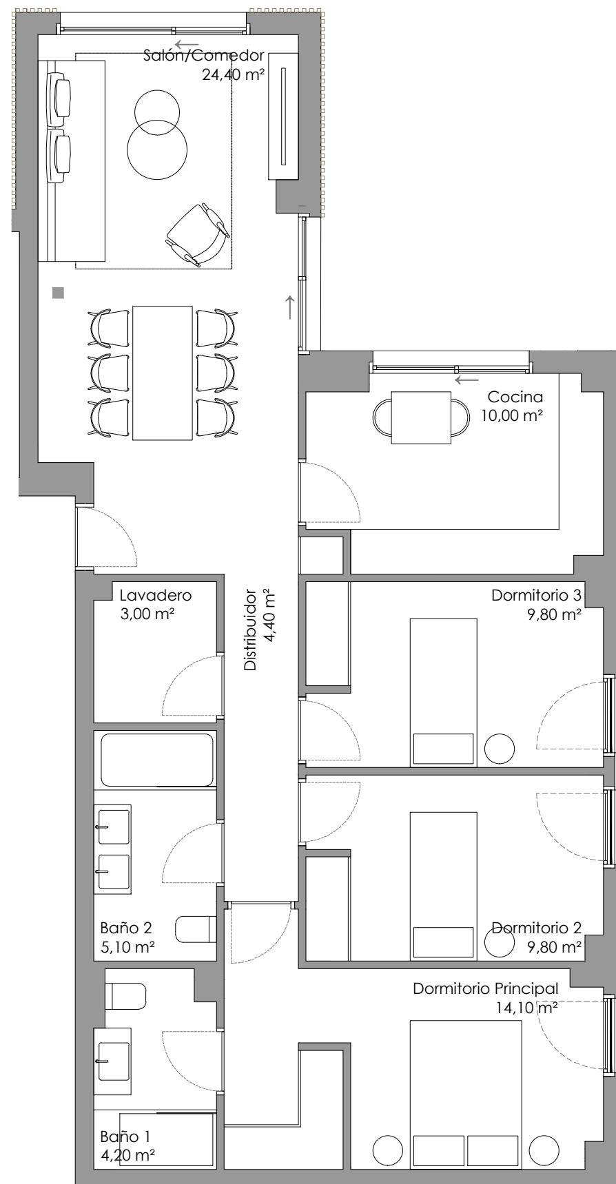
PLANTA DE VIVIENDA INTERIOR
