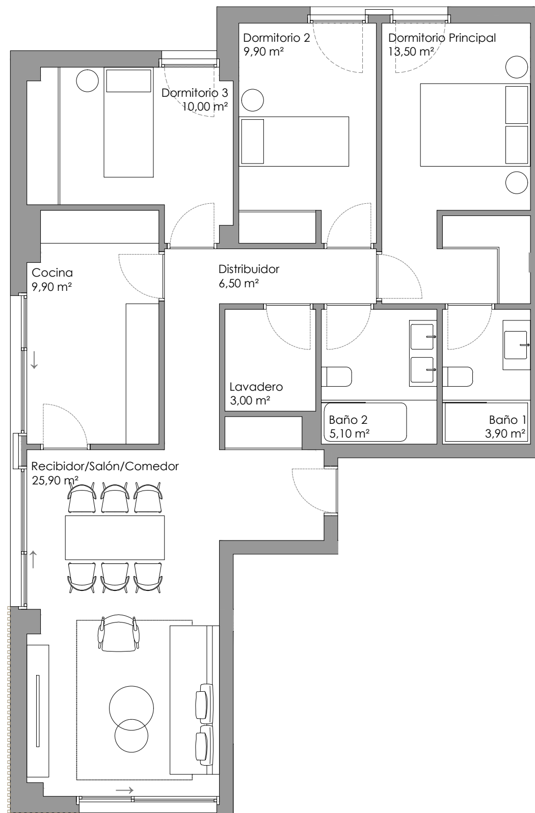
PLANTA DE VIVIENDA INTERIOR
