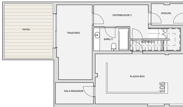
PLANTA SÓTANO
