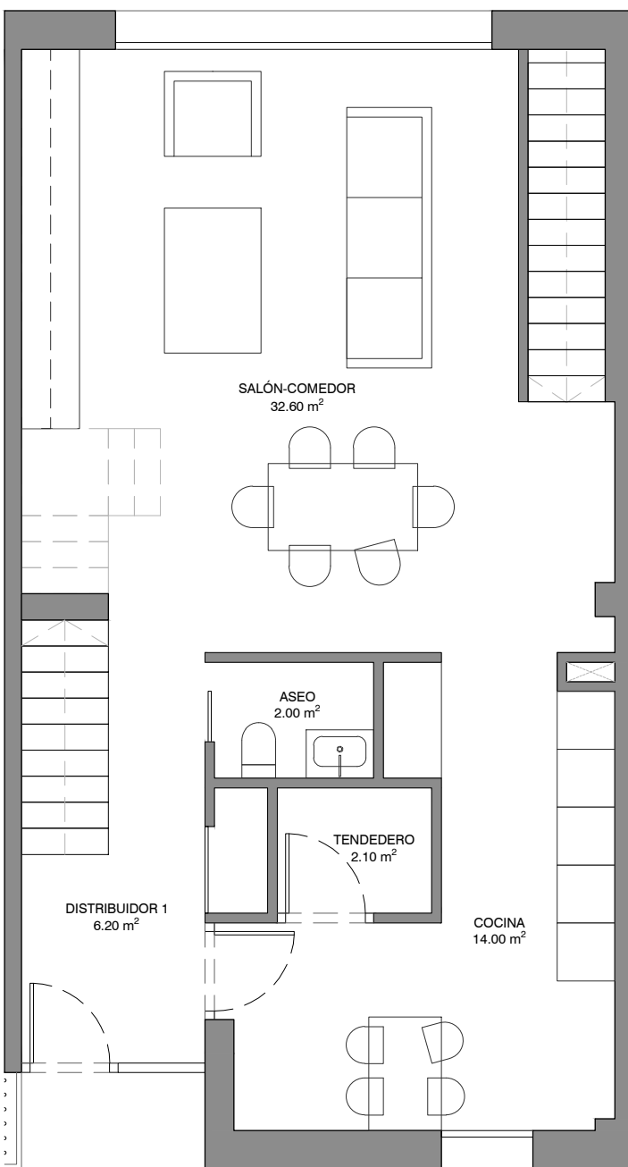
PLANTA BAJA
