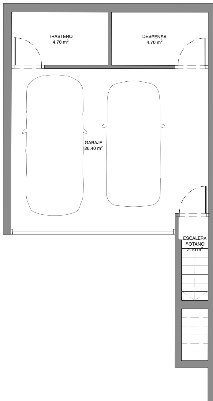
PLANTA SÓTANO
