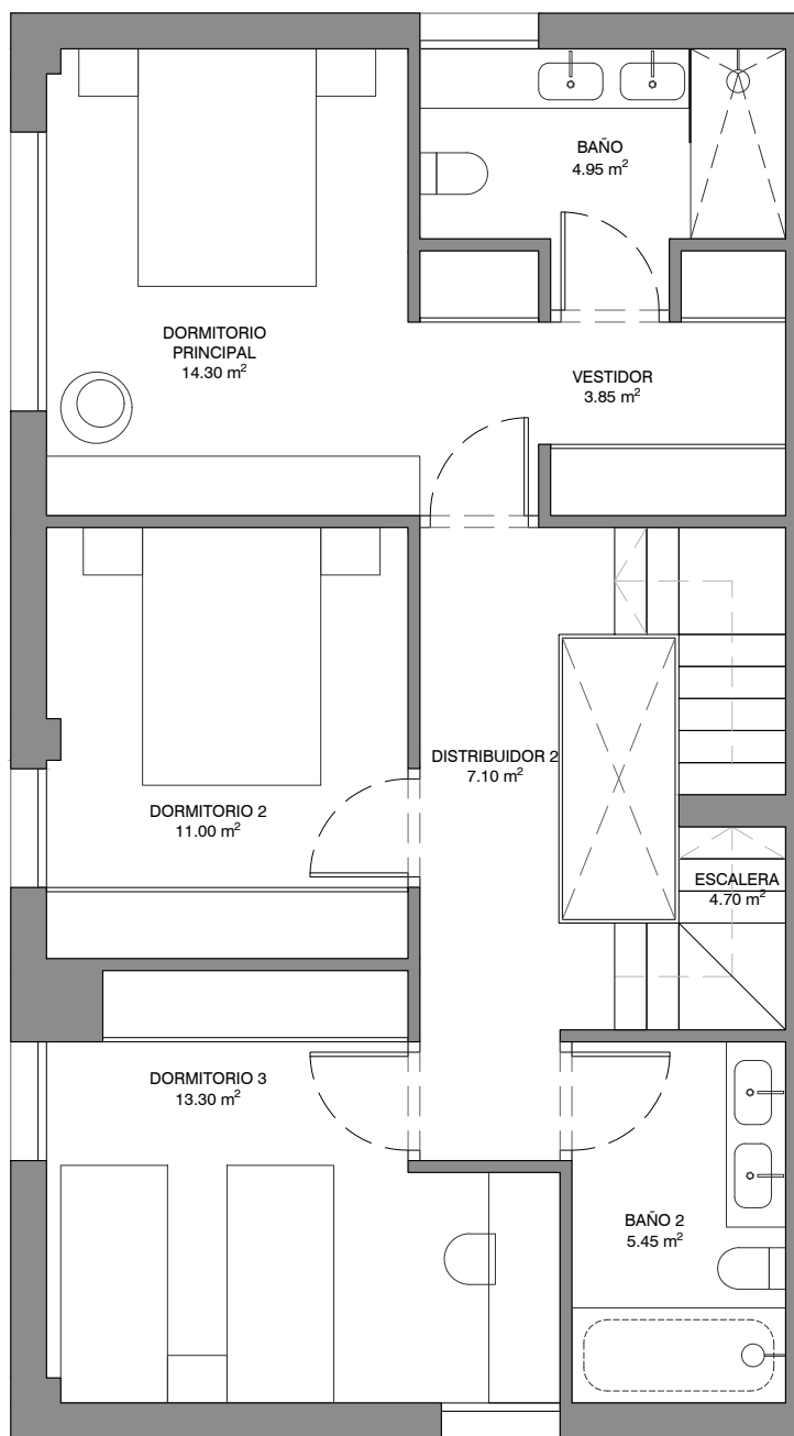
PLANTA PRIMERA
