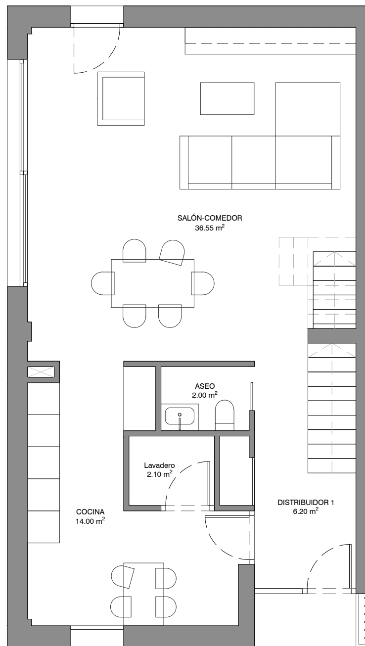
PLANTA BAJA
