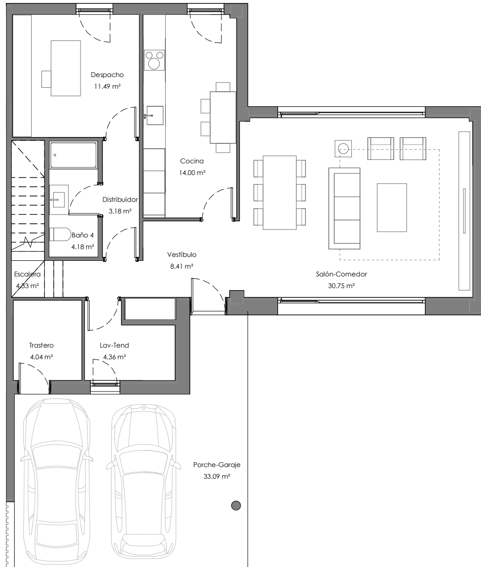
PLANTA BAJA
